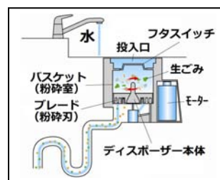
▲ディスポーザーの仕組み
